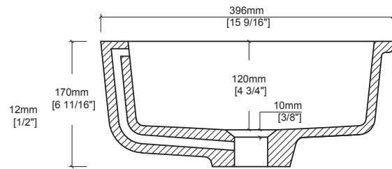
B-B
