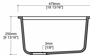
B-B
